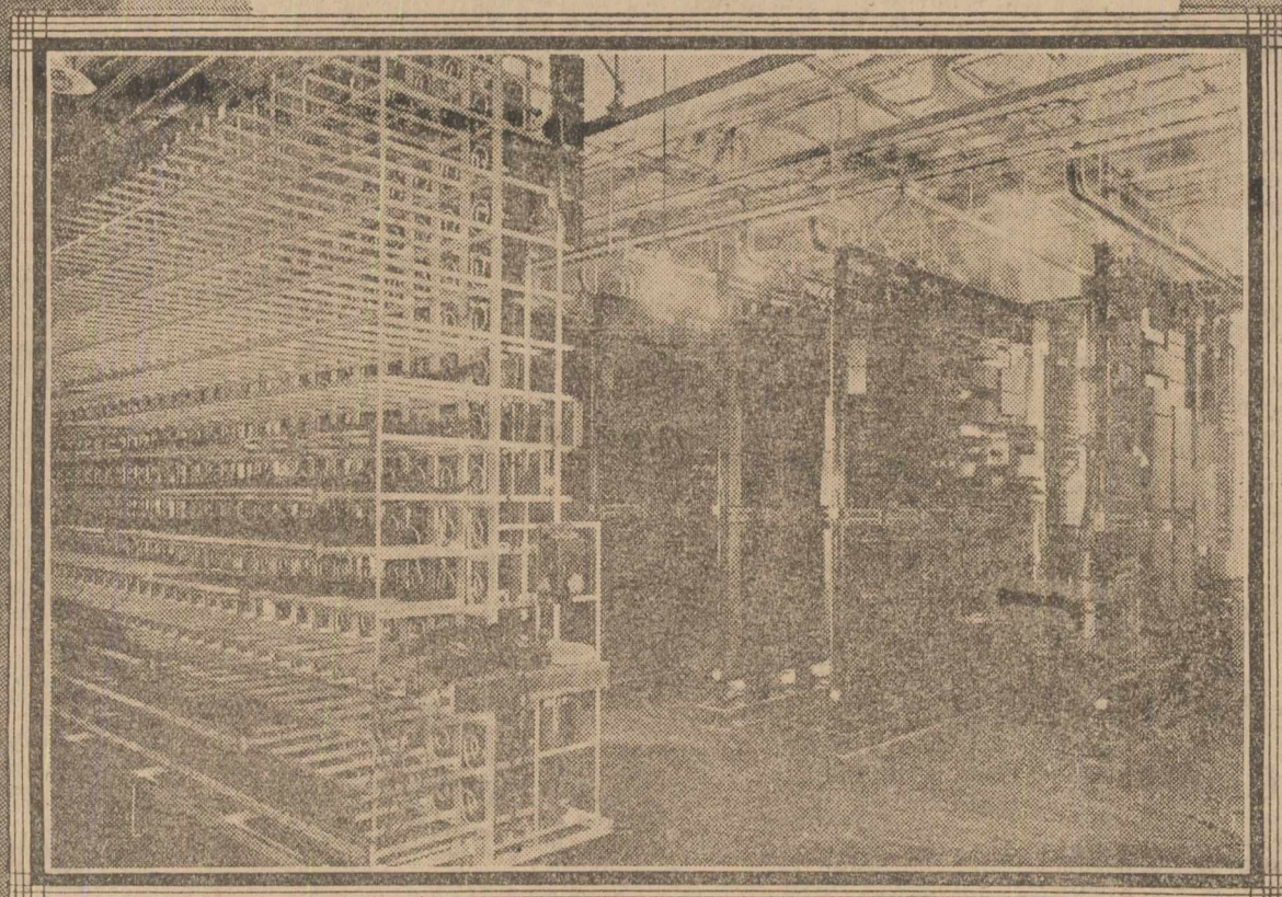
↑ CURENȚII purtători și amplificatori fac audia convorbirilor cât mai clară.
