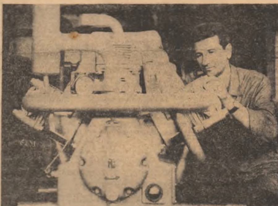
Colectivul Uzinei „Timpuri Noi” din Capitală a început fabricarea de serie a electrocompresoarelor de aer, tip 2 WC2, folosite la sistemul de frînă de la locomotiva electrică. În fotografie: controlorul de calitate Gheorghe Dobre, efectuînd recepția finală la noul electrocompresor de aer
