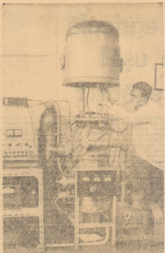
Instalația de depuneri metalice prin evaporare în vid de la Institutul de fizică atomică
