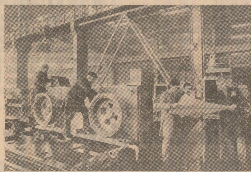
În secția utilaj complex a întreprinderii ploieștene „1 Mai” se montează un grup de motopompe. Foto: E. Dichiscanu
