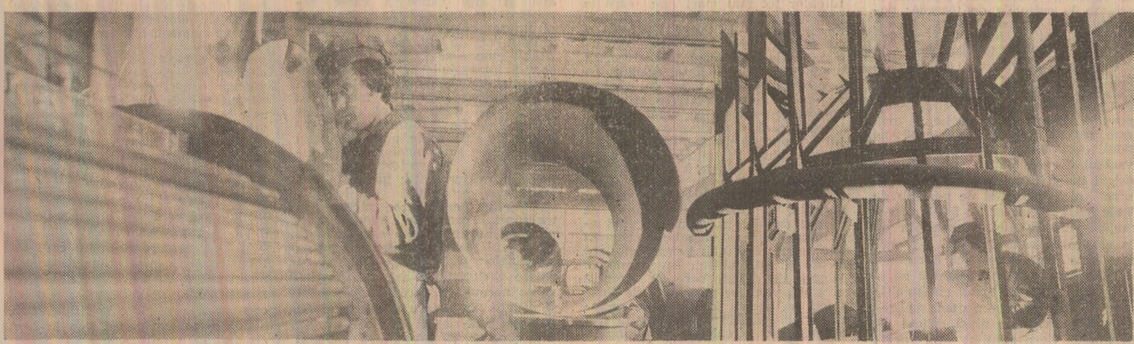
Întreprinderea de utilități tehnologice din Buzău. Aspect din secția cazangeriei grea, unde se montează subansamble pentru instalații necesare industriei nucleare petrochimice. Cea din imagine are ca beneficiar Combinatul petrochimic din Pitești. Muncitorii și specialiștii de aici s-au angajat ca print-o muncă susținută să livreze echipamentul în devans. Foto: E. Dichiseanu
