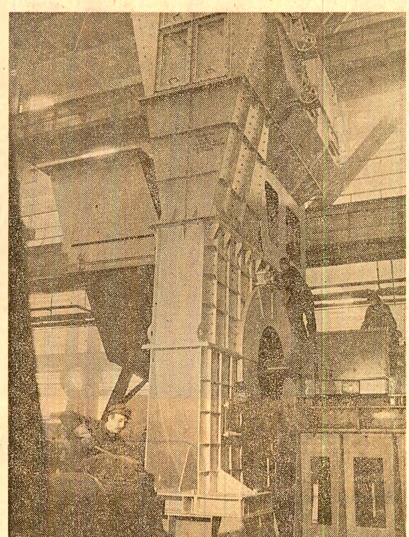
La întreprinderea „Vulcan” din Capitală, în secția roto-agregate s-a produs de curind prima moară-ventilator pentru cărbune cu o capacitate de măcinare de 50 tone pe oră, destinată termocentralei Ispolito. Este o construcție de tip nou, realizată pentru prima dată la noi în țară, cu performanțe superioare față de morile cu ciocane fabricate până acum. În fotografie: pregătirea instalației pentru probele de control pe stand
