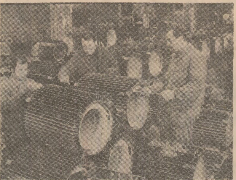
În secția a II-a montaj, de la Întreprinderea de mașini electrice din București, se lucrează la un nou lot de motoare destinate exportului. Foto: M. Alexe
