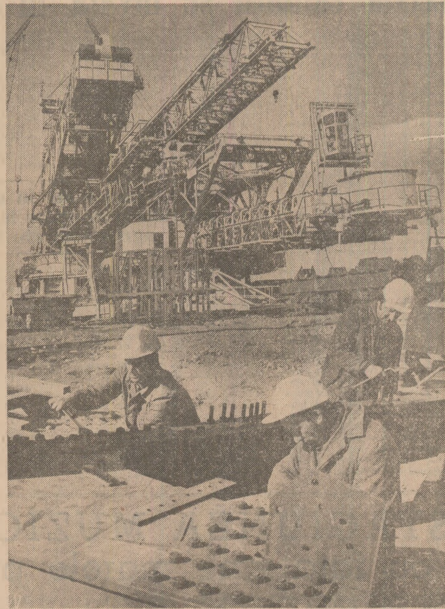
O UZINĂ... PE ȘENILE — așa poate fi numit acest excavator gigat cu rotor, de construcție românească, a cărui montare, în carierele de la Husnicioara, se apropie de sfîrșit
