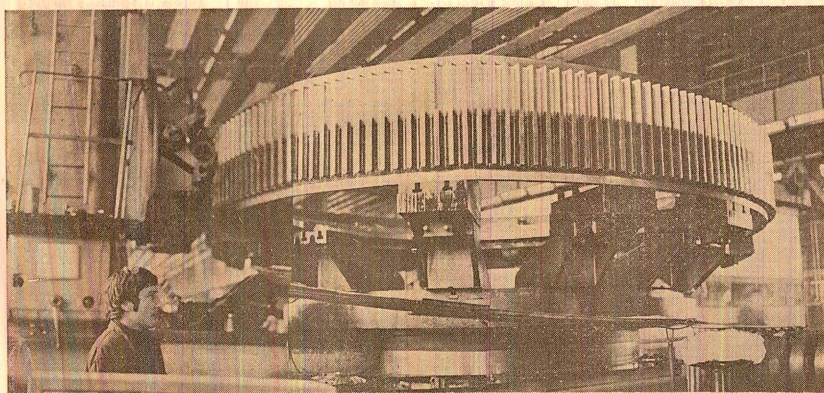
La Întreprinderea de mașini grele București se derulează zilnic secvențe de muncă tenace pentru realizarea unor produse de înaltă tehnicitate și de mare importanță pentru economia națională. În fotografia noastră, aspect din secția a III-a mecanică, unde, între altele, se execută uriașe roți dințate, necesare industriei cimentului
