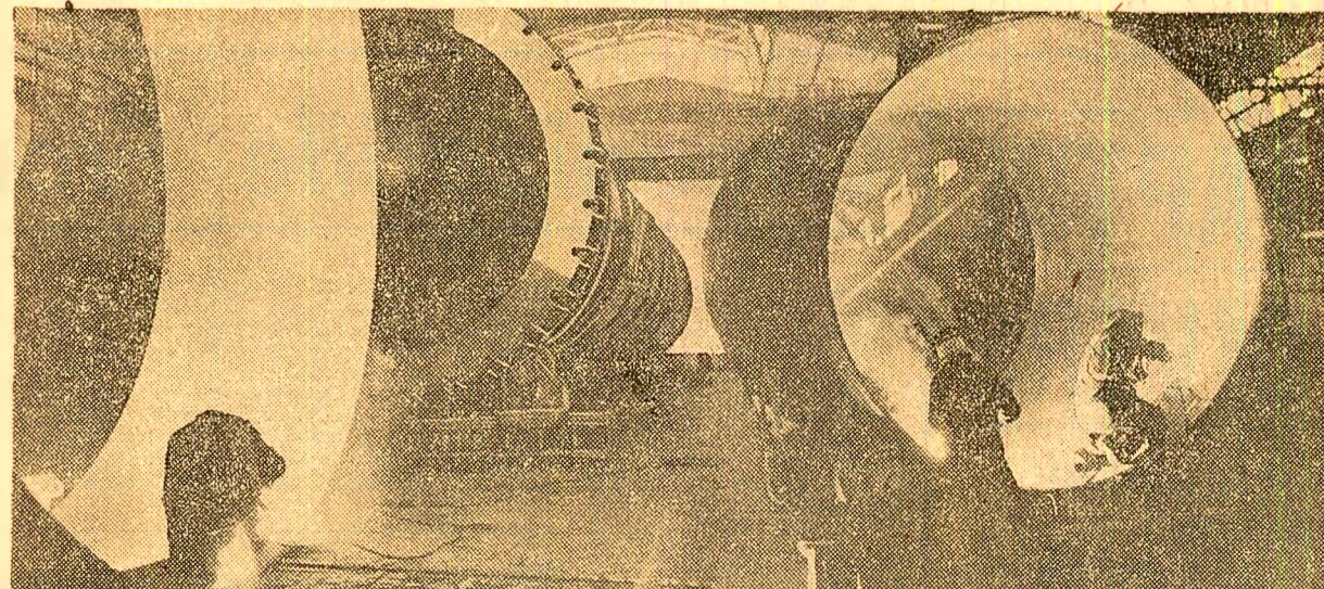
În prima zi de muncă a anului 1980 la întreprinderea de utilaj chimic „Grivița roșie” Foto: S. Cristian
