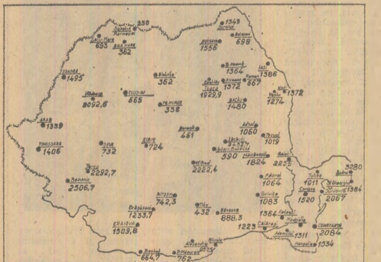
Frecvența anuală a vîntului: cifrele indică numărul mediu de ore. Prezentăm harta cu viteze ale vîntului cuprinse între 6 și 8 m pe secundă, deoarece parametrii instalațiilor pentru conversia energiei vîntului în alte forme de energie sînt calculați la viteza standard a vîntului de 8 m pe secundă
