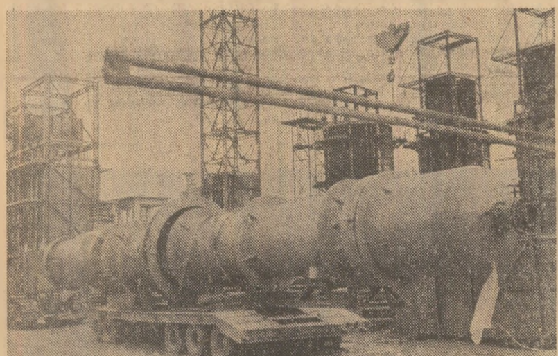
În ultima lună, la cele opt instalații ale rafinării Combinatului petrochimic de la Midia-Năvodari s-au montat peste 800 tone utilaje tehnologice. În timp ce o coloană sosită pe șantier este preluată de montori (fotografia din stînga), echipa condusă de Ion Rotaru pregătește ridicarea unei noi estacade (fotografia din dreapta)
