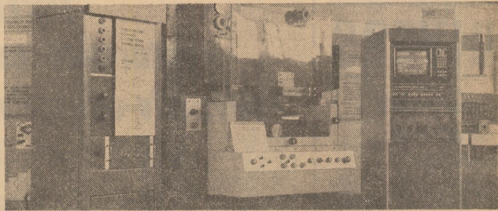
Prin MAȘINA DE PRELUCRAT PRIN ELECTROEROZIUNE CU ELECTROD FILIFORM ȘI COMANDA NUMERICĂ, utilizată pentru decupări în metale dure și extradure, la fabricarea de matrițe, ștanțe, piese complexe, industria constructoare de mașini beneficiază de o nouă tehnologie menită să ducă la creșterea productivității muncii și a calității produselor. Acest tip de mașină a fost realizat de specialiștii de la Institutul de creație științifică și proiectare tehnologică pentru construcții de mașini, Institutul de automatizări și Institutul de cercetări și proiectări electrotehnice
