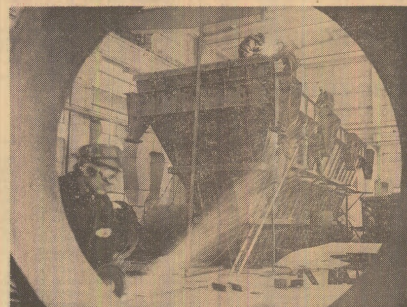
Întreprinderea de utlaj chimic din Goești. În secția cazangerie se lucrează în ritm intens la execuția unei instalații pentru industria chimică
