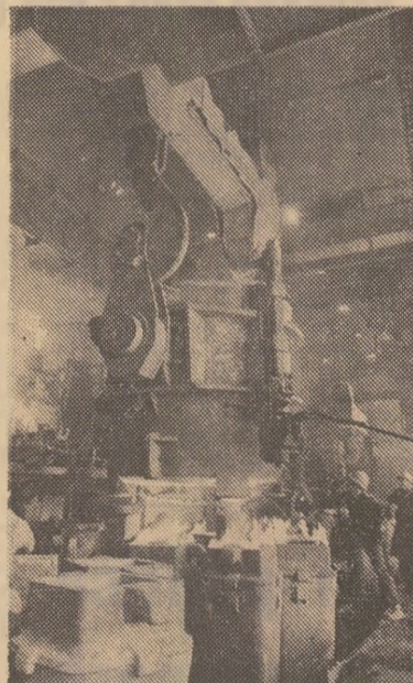
Combinatul de oțeluri speciale din Tîrgoviște. Se elaborează o nouă șărită la oțelăria nr. 2
