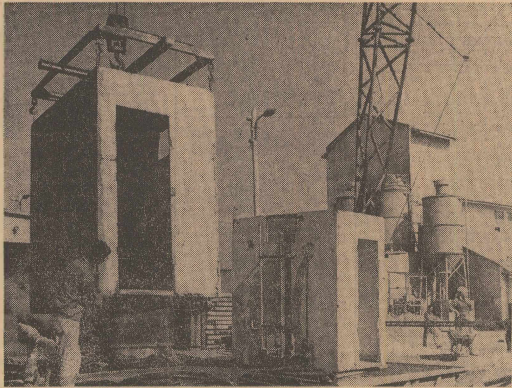
O modernă linie de fabricație la una din marile uzine de case „Granitul”. La capătul acestei linii, paralelipipedicele de beton devin
