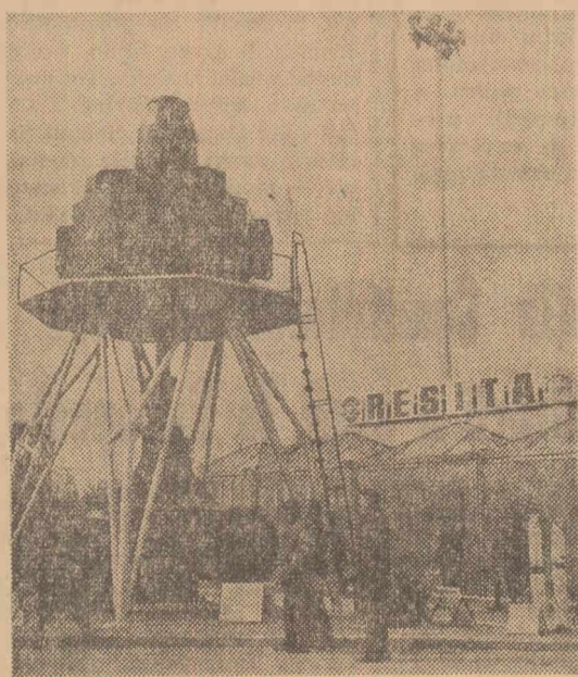
Grupul de uzine Reșița expune o gamă largă de agregate de înalt nivel tehnic. Dintre acestea se remarcă și motorul vertical de 3150 kW, cuplat cu o puternică pompă cu un debit de 25.500 m.c. pe oră, realizare a uzinei de specialitate din București
