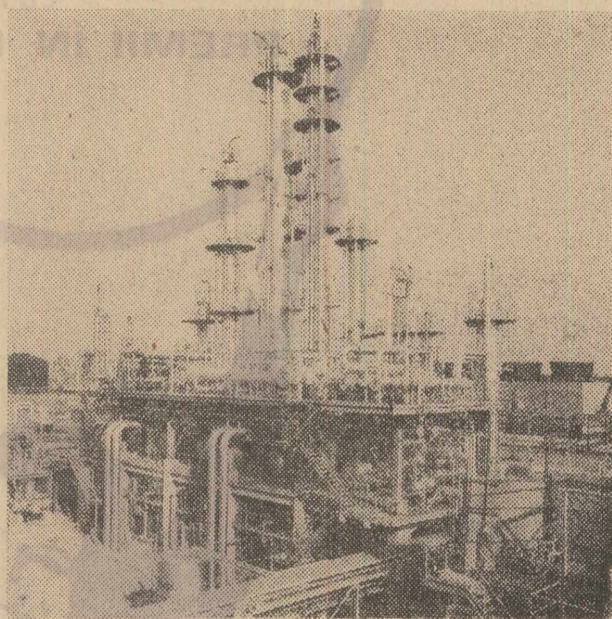
Instalație de clorură de vinil
