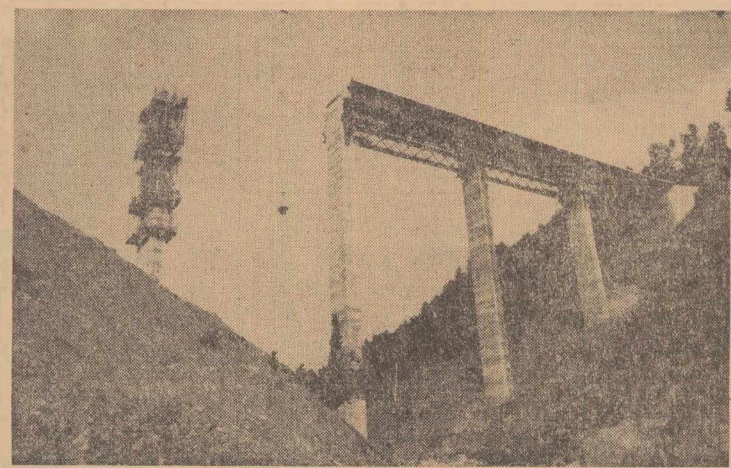
La numai 1 000 metri depărtare de barajul Paltinu se profilează silueta zveltă a unui alt obiectiv menit să asigure traversarea viitorului lac de acumulare. Este vorba de podul-viaduct Păltinoasa, operă a constructorilor de la Întreprinderea de Construcții Forestiere Buzău — șanțierul Sinaia.
