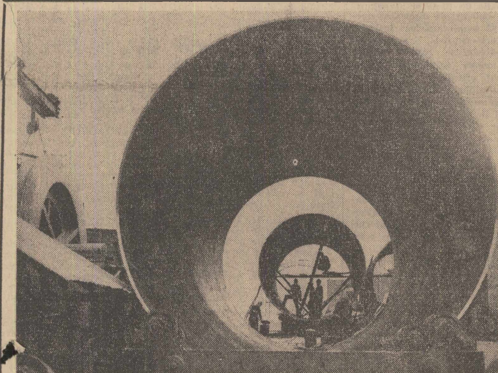
Lucrări de montaj a virolole la punctul Castelul de echilibru
