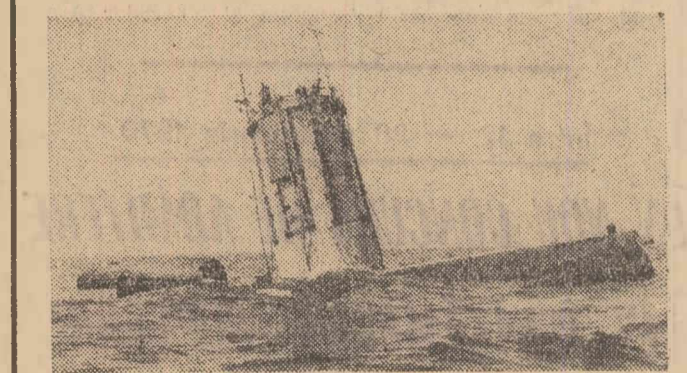
În apropierea fărâmurilor engleze, la Beachy Head, a fost instalat un nou far de semnalizare pentru nave. Construit din beton și avînd o greutate de 4.000 tone, farul are pe acoperiș, o platformă pentru aterizarea elicopterelor. Semnalele luminoase transmise de acest far vor putea fi recepționate pînă la o depărtare de 46 de mile (o milă marină = 1852 metri). În imagine — aspect din timpul transportării farului spre locul de fizare
