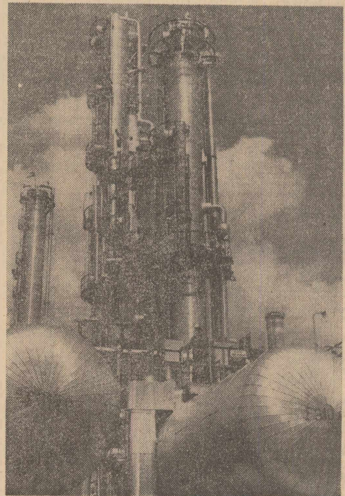
Un aspect de la citadela petrochimică românească, rod al metamorfozei socialiste: înăuntrul combinat petrochimic din Pitești
