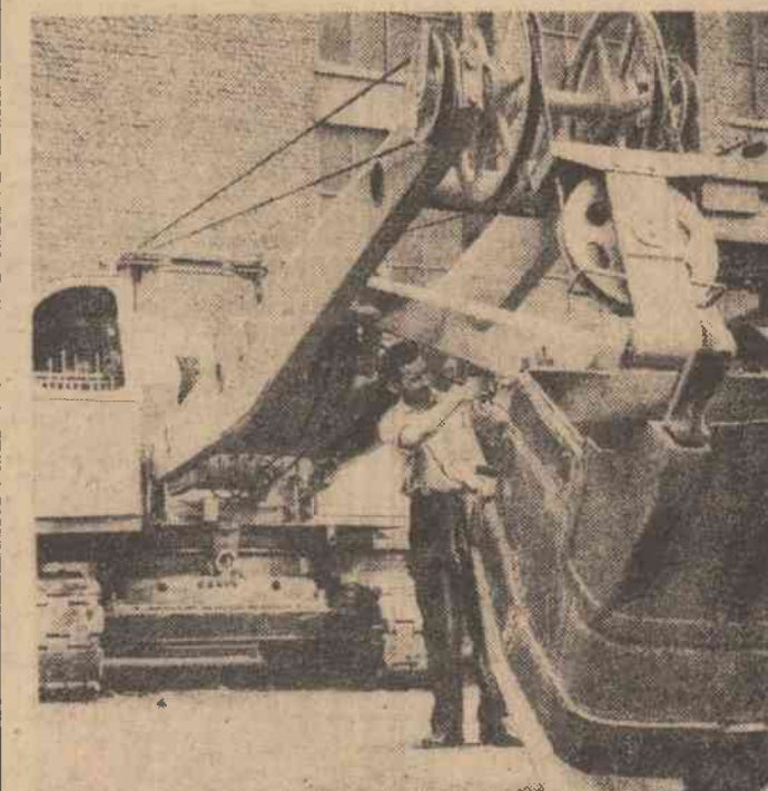
Noul tip de excavator de 0,6 m.c. aflat în probe finale la uzina „Progresul” din Brăila
