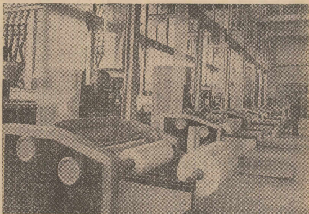
La Uzina de prelucrare a maselor plastice din Buzău a intrat în acest an în producție o nouă secție: cea de polietilenă cu o capacitate de producție de 60 tone în 24 ore. Parte din produsele realizate în cadrul acestei secții sînt destinate exportului pe bază de contracte cu un număr de circa 8 țări. În clișeu: Aspect din cadrul noii secții de polietilenă
