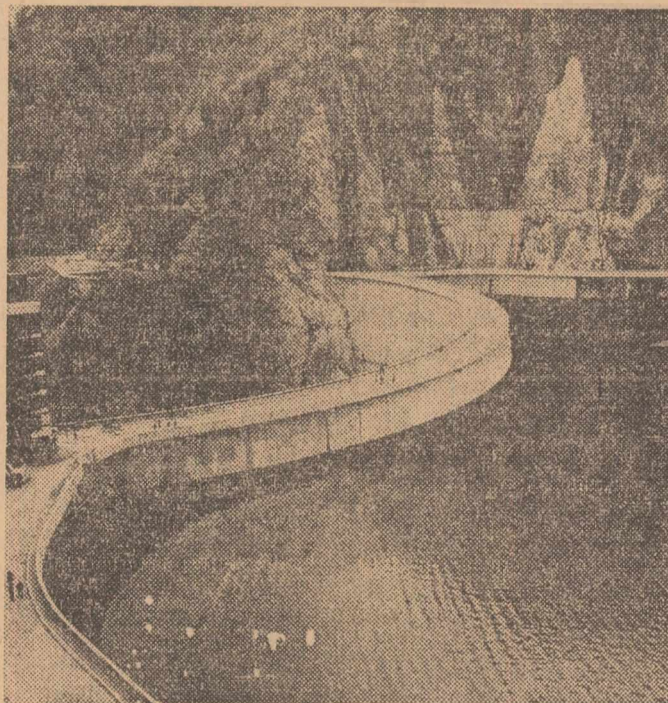
Barajul hidrocentralei de pe Argeș
