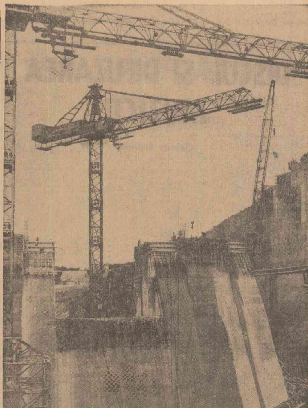
Zilele acestea constructorii de pe șantierul nr. 2 al grupului I.C.H. „Porțile de Fier” au turnat în tronsonul românesc al marelui baraj de pe Dunăre cel de al 167 000-lea metru cub de beton. În curînd ei vor atinge jumătatea din cantitatea ce urmează să se toarne la construcția din partea românească a barajului. În fotografie: aspect din timpul lucrărilor de betonare la barajul sistemului hidroenergetic și de navigație „Porțile de Fier”
