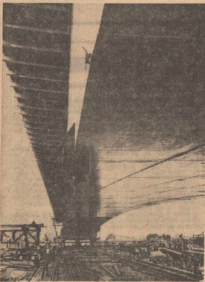
Tablierul a fost lansat la apă pe șlepur
