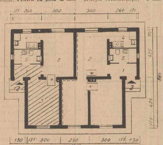
Institutul pentru studii și proiectări de sistematizare, arhitectură și tipizare a realizat un album cu proiecte pentru locuințe tip în mediul urban și rural, realizabile în etape. Albumul va fi difuzat zilele acestea. Una din variante — cea de mai sus — prezintă două gospodării rurale cuplate printr-un perete comun, trasat în schița din stînga printr-o linie punctată. Schița înfățișează distribuția încăperilor în cadrul celor două gospodării. Zona hășurată indică varianta unei prime etape în construcție. Locuințele sînt compuse din două și respectiv trei camere și dependințe. În clișeu din dreapta: vedere exterioară a clădirilor.
