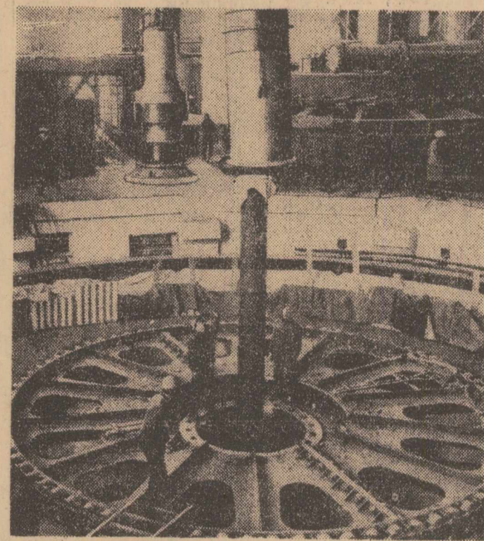
Pentru montarea rotorului primului generator, de la Porțile de Fier, au fost necesare cinci luni. În structura uriașă, cu un diametru de 14 m, și cîntărind nu mai puțin de 650.000 kg, au intrat 11.000 de piese diferite, produse în întreprinderi din întreaga țară. În imagine: un aspect din faza de montaj Foto: MIHAI POPESCU
