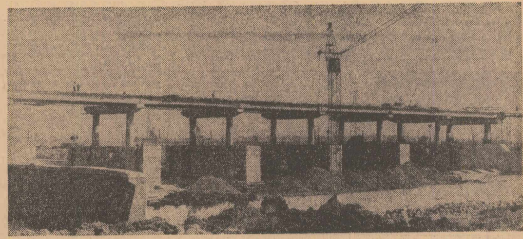
Construcții Centralei termoelectrice Rogojel au încheiat lucrările de betonare a barajului de retenție de pe Iiu, construit în avalul acumulării de la Rovinari. Barajul, aflat acum în stadiul montajului echipamentelor hidromecanice, a fost proiectat pentru sursa de apă industrială a centralei termoelectrice. Este amplasat de-a curmezișul noii albie a Jiului, canalizat în cadrul amenajărilor complexe executate în vederea exploatării imenselor zăcă-minte de lignit din acest mare bazin carbonifer. Este al treilea baraj de pe cursul mediu și inferior al Jiului, după obiectivele de același gen construite la termocentralele Craiova și acumularea Rovinari. În fotografie: vedere generală a barajului de la Rogojel.
