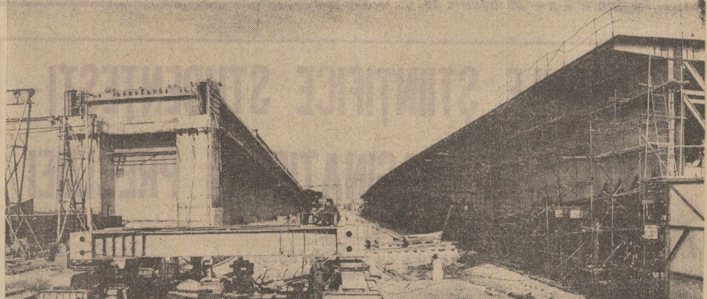
Imaginea de mai sus a fost luată de pe malul de la Giurgeni. În stînga se profilează construcția din beton a viaductului, iar în dreapta primul bloc al tablierului metalic pregătit pentru lansare pe pilonii din albia fluviului
