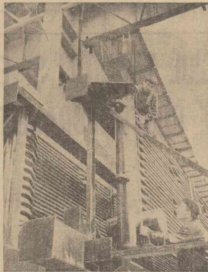
La Uzinele „Vulcan” din Capitală a început de curînd construcția primelor subansamble ale cazanului de 1.000 tone abur pe oră. În faza finală, cazanul va avea o înălțime de circa 100 m și un consum de 1.035 tone lignit în 24 de ore și va alimenta o turbină de 330 megawați. Realizarea acestui mare cazan dovedește creșterea gradului de maturitate al acestei mari uzine bucureștene. În clișeu: Aspect din cadrul secției de țevărie a uzinelor „Vulcan” unde se lucrează la asamblarea unui lot de instalații destinate termoficării. Foto: AGERPRES
