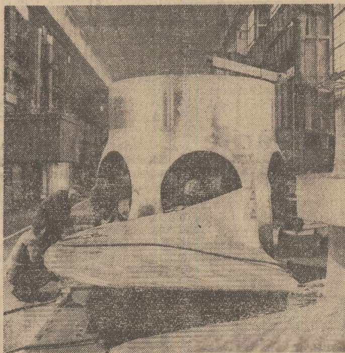
La Uzina de construcții de mașini din Roșia se fabrică o bună parte din hidroagregatele destinate marelui șantier hidroenergetic și de navigație de la Porțile de Fier. În clișeu: Aspect din secția de mecanică grea
