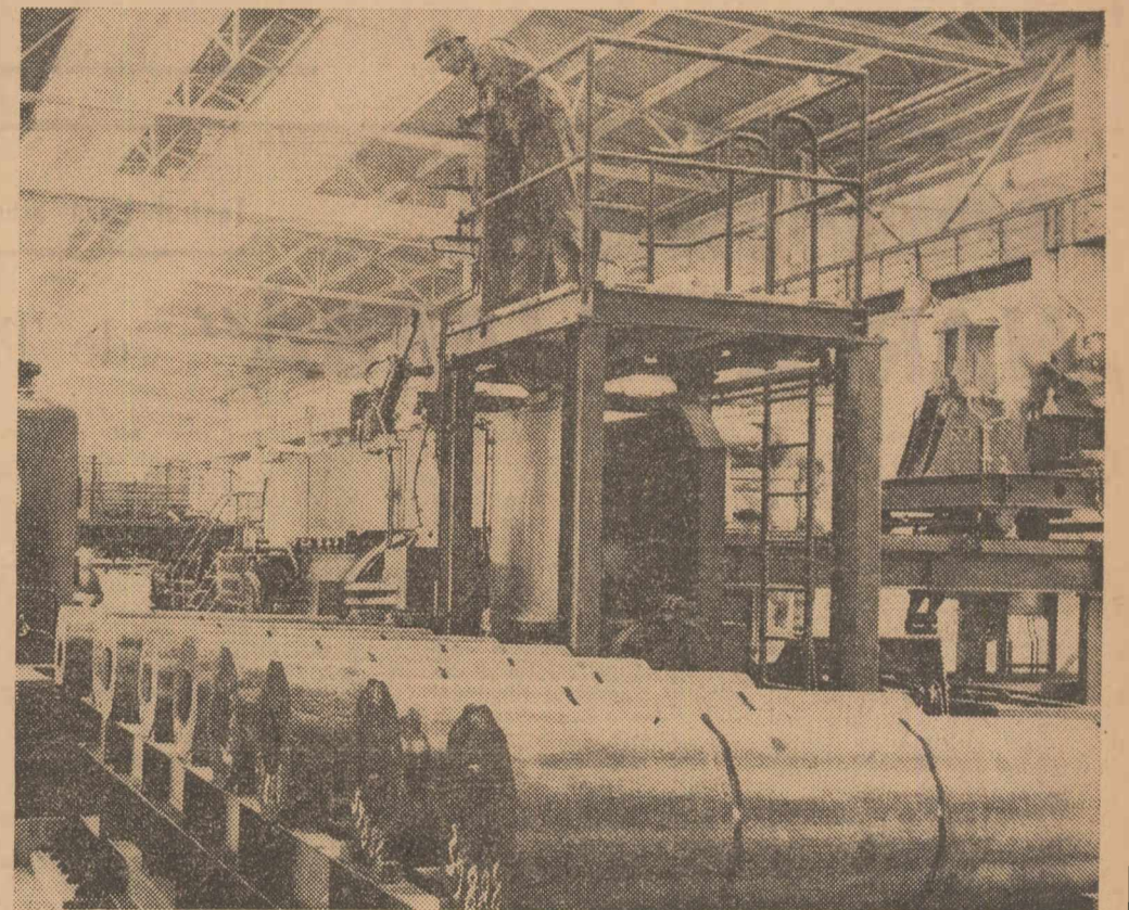
Din aceste lingouri de oțel, grele de peste 2 000 de kilograme și cu un diametru de circa jumătate de metru, spargătorul de blocuri hidraulic detașează în cîteva secunde calupul de metal din care puțin mai tîrziu, va lua naștere o roată de vagon
