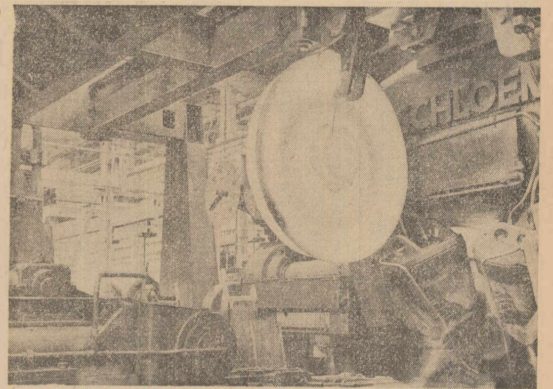
Acum câteva zile, anunțăm realizarea, la Fabrica de oșii și boghiuri din Balș, județul Olt, a primei roți monobloc. Fotografia de față a imortalizat clipa în care, după ce a fost prelucrată în modernul laminor (de laminare în poziție verticală fără gaură), roata este purtată cu ajutorul unor clesți speciali spre presa de 2.000 de tone, un alt utilaj important al fluxului tehnologic, unde urmează să se facă ultimele operații: ondulară discului și găurirea butucului.
