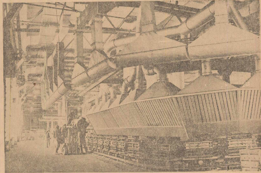
Aspect din noua turnătorie de fontă, intrată parțial în funcțiune, în cadrul Uzinei de autocamioane Brașov. După cum se poate lesne observa, condițiile de muncă ale turnătorilor sînt total schimbate față de cele de pînă acum
