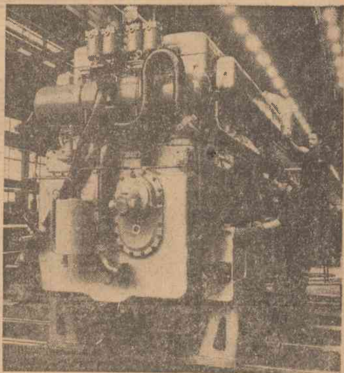
Constructorii de mașini aparținînd grupului de uzine Reșița, și-au depus sarcinile în primele două luni ale anului livrînd în plus peste 450 tone diferite mașini și utilaje pentru industria chimică și industria metalurgică, precum și motoare electrice cu o putere totală de 6 000 K.W. În clipă: Aspect din secția motoare Diesel.
