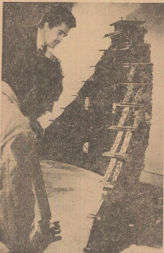
La Institutul de studii și proiectări hidroenergetice se efectuează măsurători și probe de laborator, pe machete, pentru determinarea diferiților factori ce acționează, intern sau extern, asupra barajelor sau elementelor componente. În clipă: Macheta barajului Tarnița (Lotru) supusă unor asemenea măsurători
