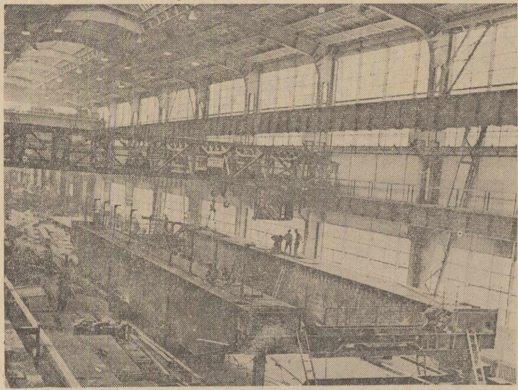
Le Uzina de construcții metalice și mașini agricole Bocșa se montează un pod rulant de 33,5 m lățime și cu o putere de ridicare de 320 tone
