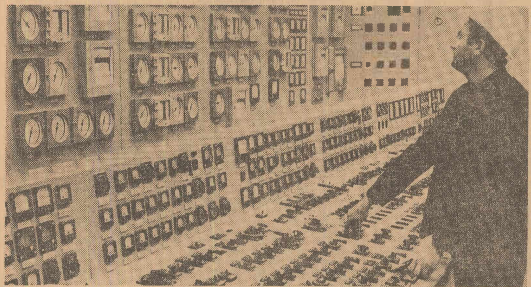
LA sfîrșitul anului trecut, amuzăm faptul că la Centrala termoelectrică de la Dava a fost conectat la rețeaua sistemului energetic național primul grup cu o putere instalată de 210 MW. În clișeu Un aspect din camera de comandă a primului grup energetic.
