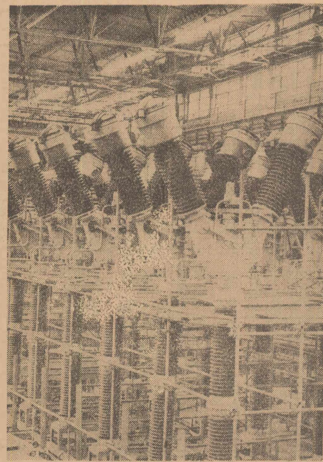
La uzinele „Electroputere”-Craiova, lucrătorii fabricii de aparatură dau viață angajamentelor luate în întrecerea socialistă. Iată un nou lot de întrerupătoare automate gata de a fi expediate beneficiarilor.
