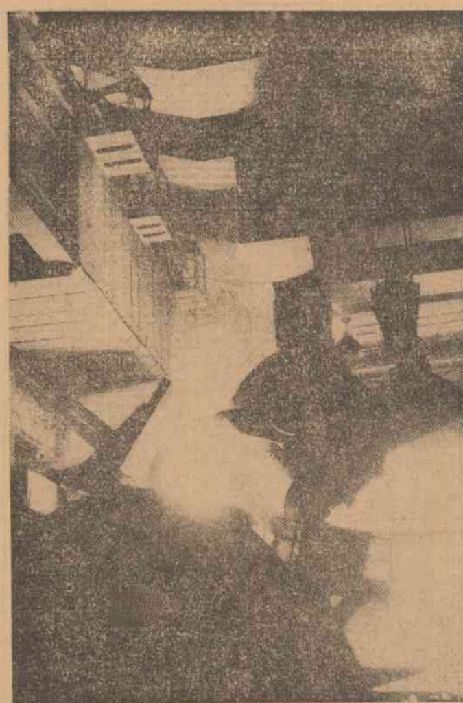
Un moment important în activitatea cotidiană a oțelărilor gălățeni — turnarea fontei în melanjor, unde va fi menținută la o anumită temperatură, pentru a alimenta convertizorul
