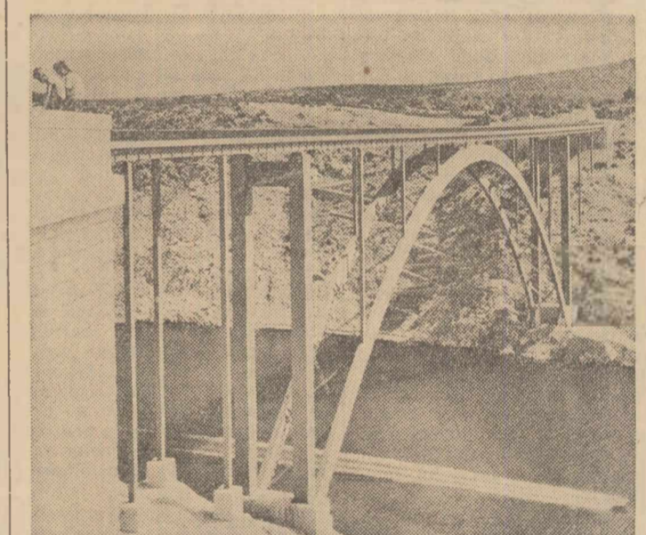
Primul pod maritim construit în Iugoslavia (imaginea de mai sus) se află în apropierea localității Šibenik și leagă între ele cele două maluri ale Golfului Marina. Considerat ca una dintre realizările remarcabile ale constructorilor de drumuri și poduri din țara vecină și prietenă, acest pod a fost proiectat și construit de specialiștii uzinei „Duro Djakovic” din Slavovski Brod, oraș cu aproximativ 30.000 de locuitori, situat la jumătatea drumului dintre Zagreb și Belgrad. Produsele acestei uzine — una dintre cele mai mari întreprinderi iugoslave în domeniul industriei construcției de mașini și echipament greu — sînt cunoscute și apreciate în întreaga țară, cit și peste hotarele ei.
