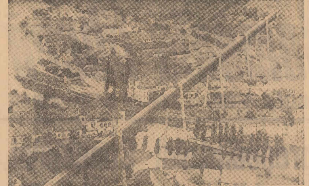
Aducînd o notă inedită în peisajul pitoresc al orașului, podul-funicular care brăzdează cerul Reșiței transportă calcarul necesar în procesul de producție al Combinatului siderurgic de pe malurile Birzavei
