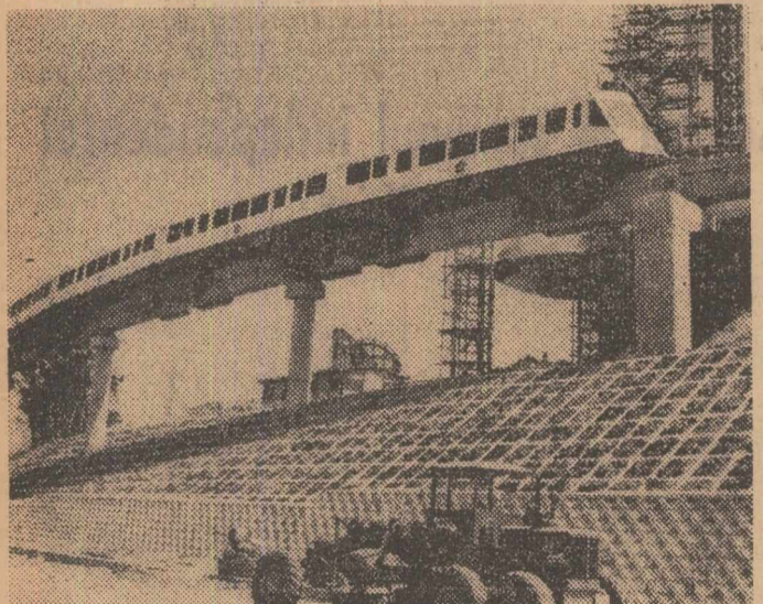
Cu câteva zile în urmă a fost terminată instalarea primului tren monorail, destinat să asigure transportul vizitatorilor viitoare expoziții mondiale, care se va deschide anul viitor la Osaka (Japonia), în timpul expoziției, vase trenuri care au cel fotografic, fiecare cu cîte patru vagoane, vor circula în continuu pe cei 4,3 km de linie ferată care înconjoară „Expo-70”.
