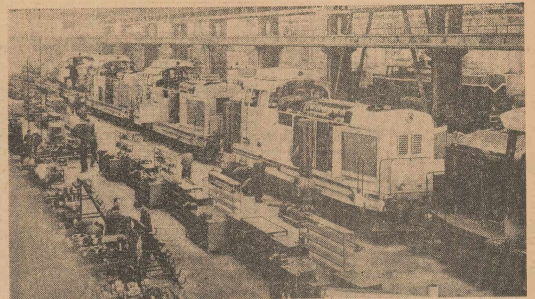
La Uzinele 23 August din Capitală se află în pregătire noi variante de locomotive. În vederea satisfacerii cerințelor beneficiarilor externi, în trimestrul I al acestui an a fost întocmit proiectul de execuție pentru locomotiva Diesel hidraulică de 450 CP cu echipament de 1 000 mm, pentru R.P. Polonă. Se află de asemenea, în curs de proiectare locomotiva Diesel hidraulică de 700 CP pentru R.P.D. Coreeană, prevăzută cu cuplă centrală automată și locomotive de 450 CP adaptate pentru țările calde, solicitate de R.A.U. În cliseu: se montează un nou lot de locomotive Diesel hidraulice de 1 250 CP.
