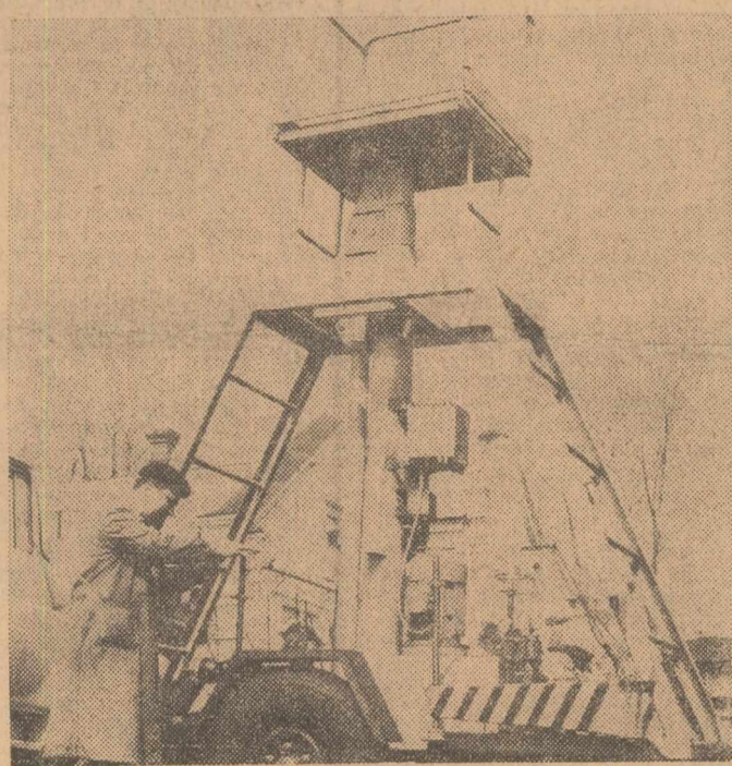
Platforma telescopică hidraulică care poate ridica o sarcină de 180 kg la o înălțime de 12 metri. Este folosită la lucrările din centralele electrice precum și în alte domenii.
