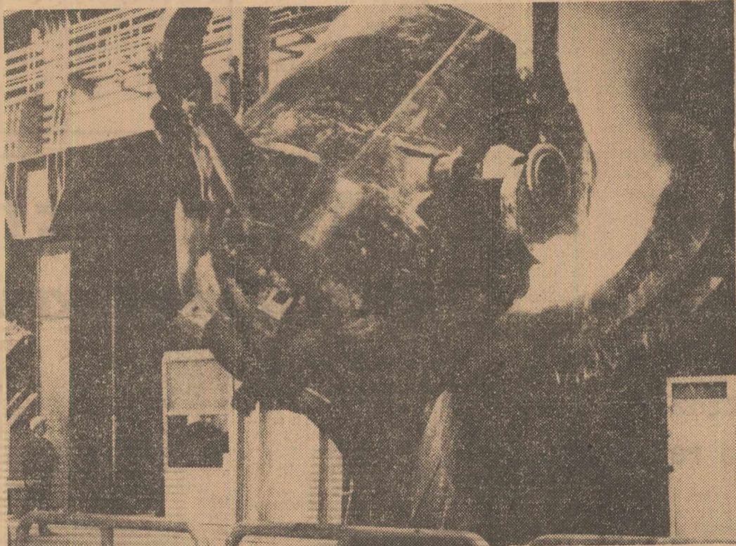
Platforma modernizării oțelării gălățene. Moment solemn: se toarnă fonta lichidă în convertizor.
