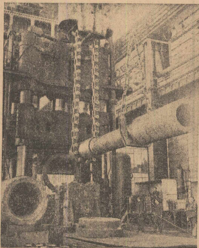
Uzina de mașini grele din București este una din marile întreprinderi producătoare de piese grele de mașini. În cliseu : Aspect din timpul forării la giganta presă de 600 tone forță a unui butuc destinat industriei constructoare de mașini
