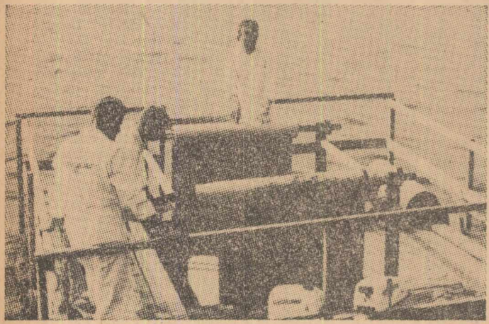
Instalația din fotografia de mai sus a fost construită după proiectul inventatului suedez Eugen Larsson și poartă numele de „sugativă de petrol”. Ea este folosită pentru combaterarea poluării apelor și acționează pe baza proprietății unei hirtii speciale — introdusă într-un lichid — de a absorbi doar substanțele petroliere
