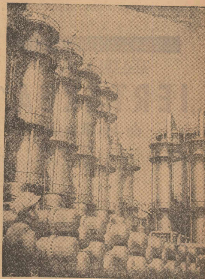
Combinatul chimic de la Craiova se înalță falnic pe plaiurile albe-negri îmbogățind peisajul industrial al țării. În cliseu: instalațiile fabricii de amoniac din cadrul combinatului craiovean
