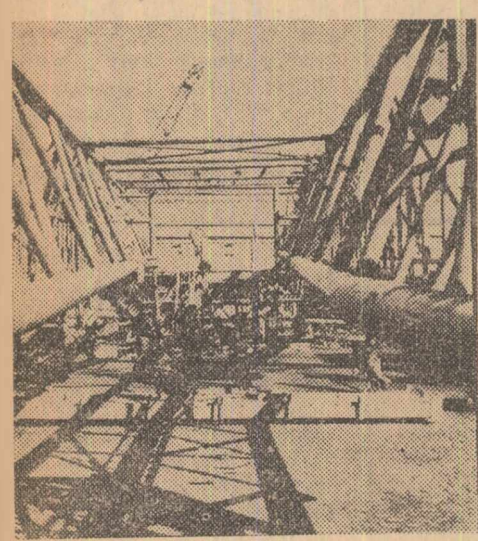
Fotografia prezintă o modernă instalație de foraj românească, realizată la Uzina „I. Mai” din Ploiești și care a fost livrată R.P. Polone în cadrul schimburilor economice româno-polone, în timpul montării ei la locul de destinație.
