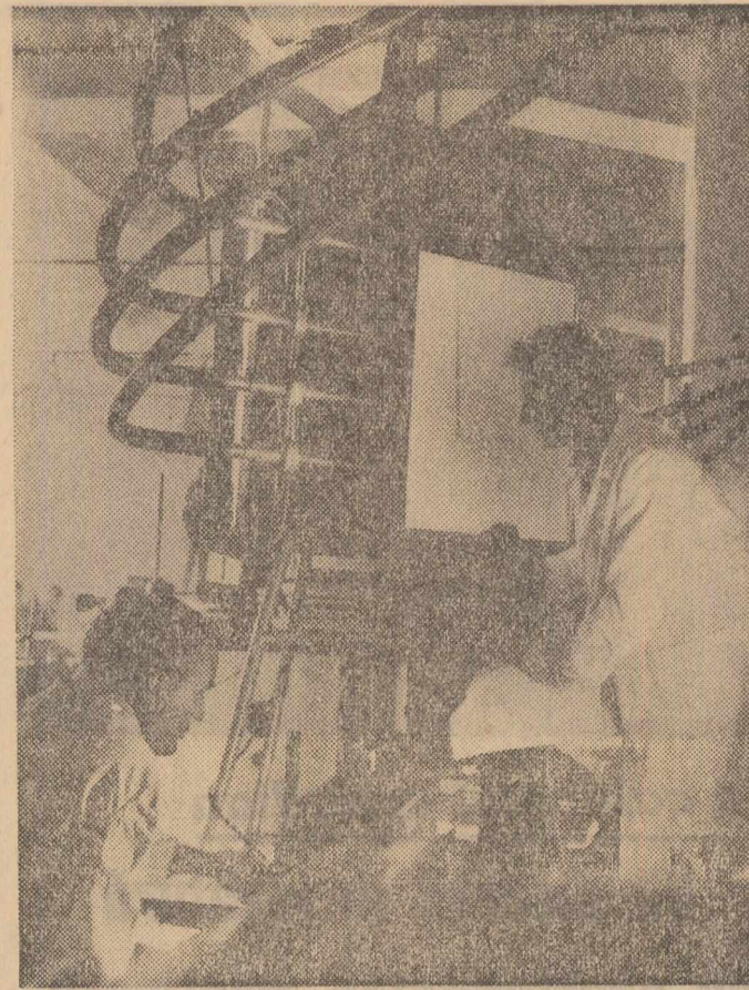
În secția hidromecanică a Institutului de mecanica fluidelor „Traian Vuia” funcționează o instalație pentru studiul mișcărilor cu viteză ce apar în diferite construcții hidraulice. Rezultatele obținute (cu caracter general) au fost recomandate I.P.A.C.H. la proiectarea și execuția diferitelor lucrări hidrotehnice. În clădire: Cercetătorul principal inginer Costel Iancu și tehnicianul Petre Vasilescu în timpul unor lucrări de studiu
