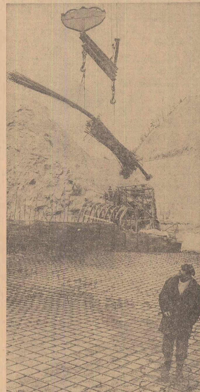
În albia Dofanei se betonează intens. Curînd la malul stîng se va atinge cota finală a barajului Palinu. De un mare ajutor constructorilor este macarava funicular instalată deasupra văii, care pe lîngă benele de beton transportă în amplasamentul dotat diverse materiale. În cîleș: un „snop” de armături coborât din înălțimi. Foto: NICU VASILE
